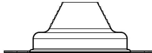
SECTION B-B SCALE 1 : 7
